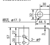
側面安裝支架
