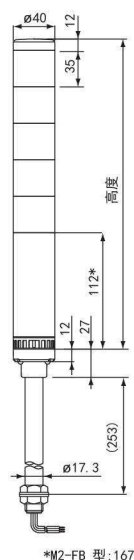
LCE 型 LCE-U 型
