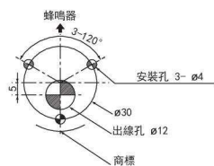
安裝尺寸
