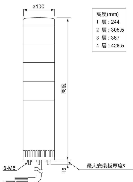
安裝尺寸
