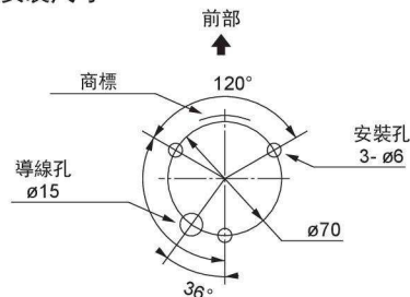
安裝尺寸
