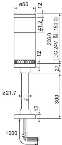
LME 型
