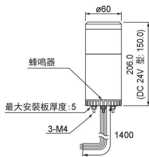
LME-W 型
