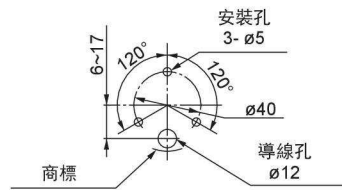
安裝尺寸
