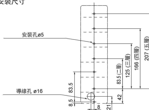
安裝尺寸
